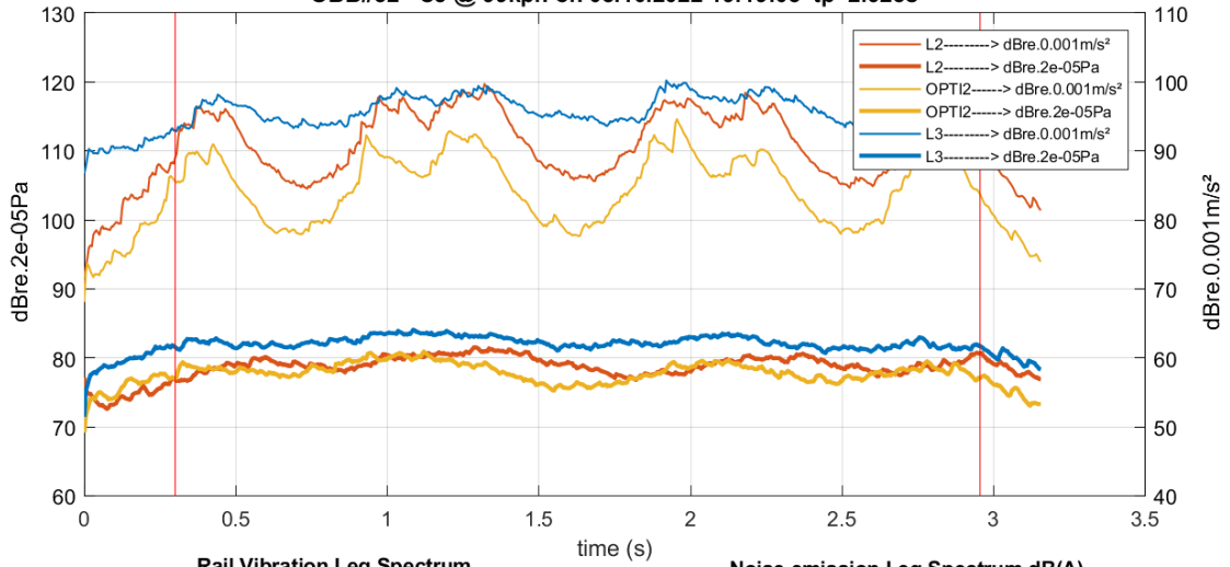
ÖBB#52 CJ @ 99kph on 08.10.2022 19:19:05 tp=2.625s
