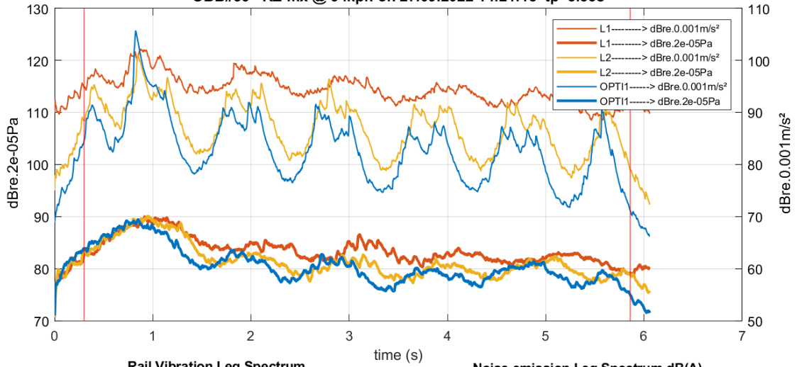
ÖBB#59 RZ-mx @ 94kph on 27.09.2022 14:21:18 tp=5.53s
