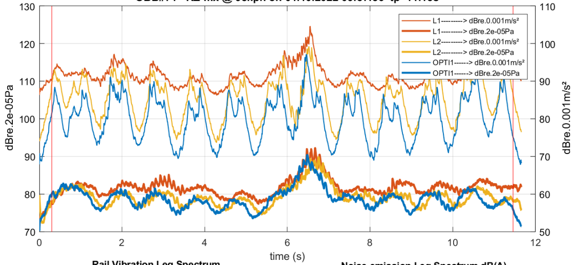
ÖBB#71 RZ-mx @ 98kph on 01.10.2022 09:57:56 tp=11.13s
