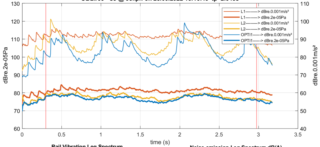
ÖBB#63 CJ @ 98kph on 28.09.2022 15:16:43 tp=2.645s
