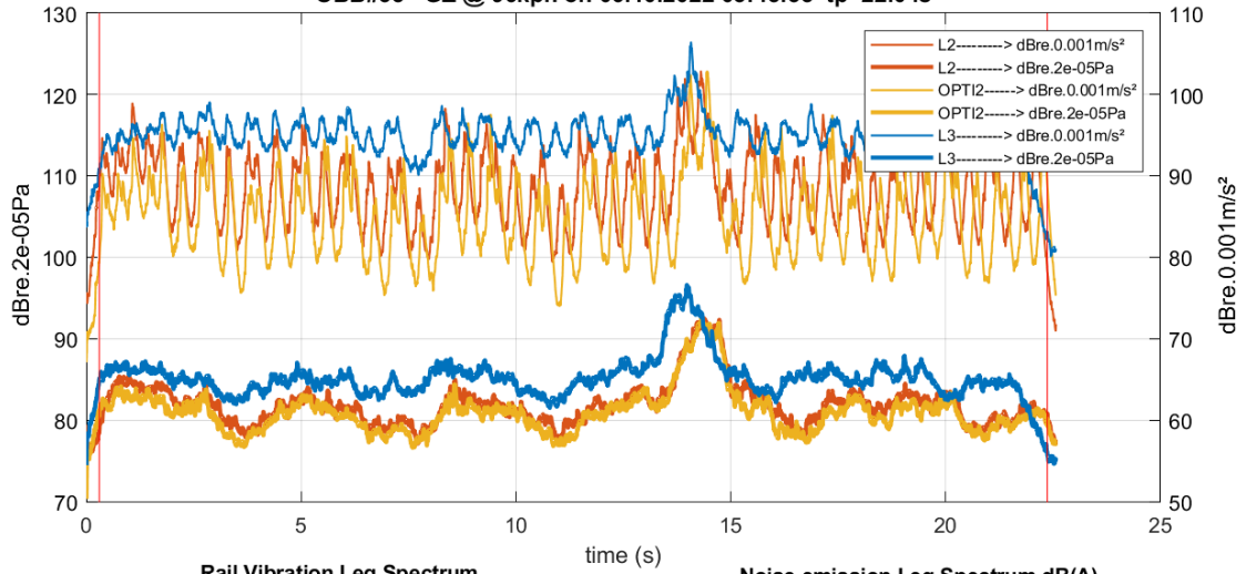
ÖBB#35 GZ @ 96kph on 06.10.2022 03:45:35 tp=22.04s
