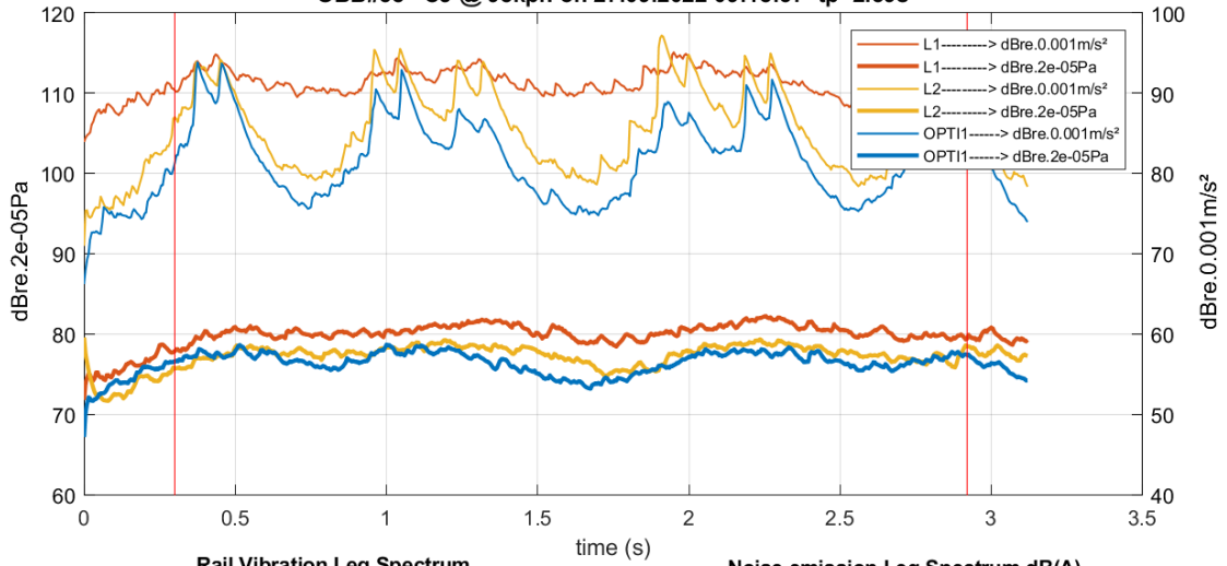
ÖBB#58 CJ @ 98kph on 27.09.2022 09:18:37 tp=2.59s
